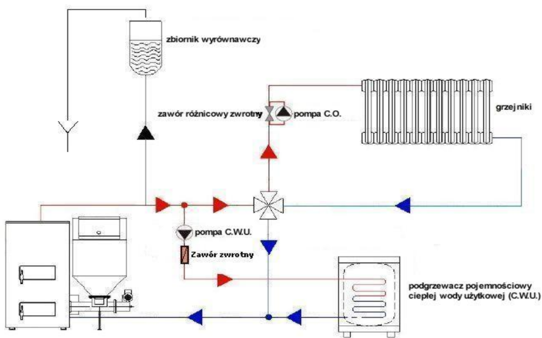
Schemat ideowy instalacji z zaworem czterodrożnym.
