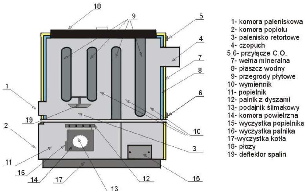
Przekrój kotła typu ECO LUX 18-25kW
