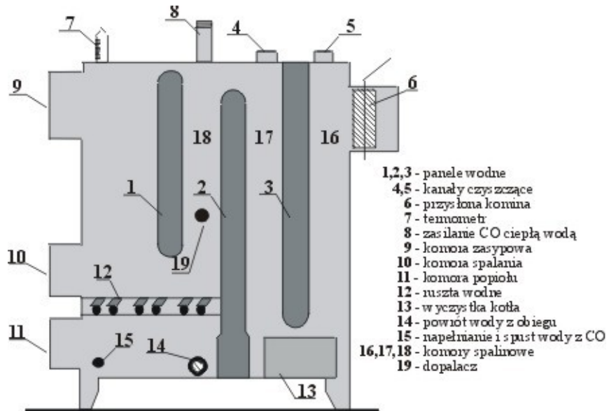
Przekrój kotła
