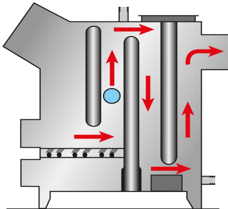
Przebieg spalin
